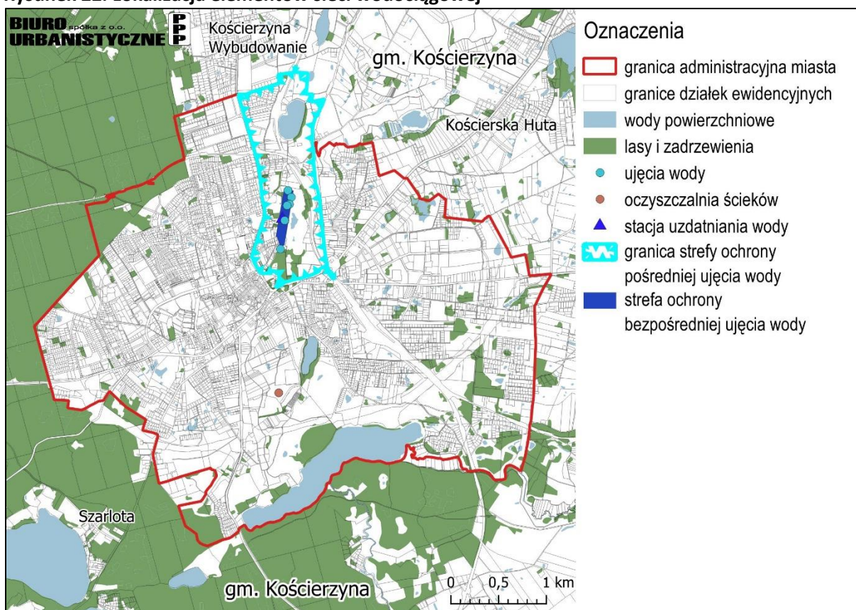
Rysunek 22. Lokalizacja elementów sieci wodociągowej
